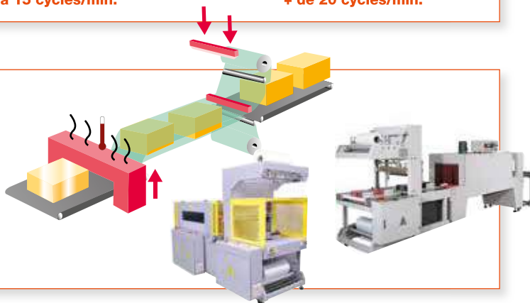
Soudeuse semi-automatique et tunnel 8 à 15 cycles/min.
